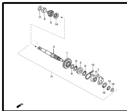
E-11 EJE CRANK
