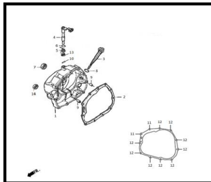
E-7 CARCAZAS CENTRALES
