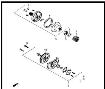
E-9 CAJA CAMBIOS
