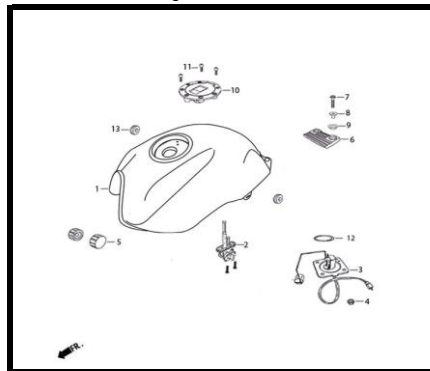
F-10 TANQUE COMBUSTIBLE
