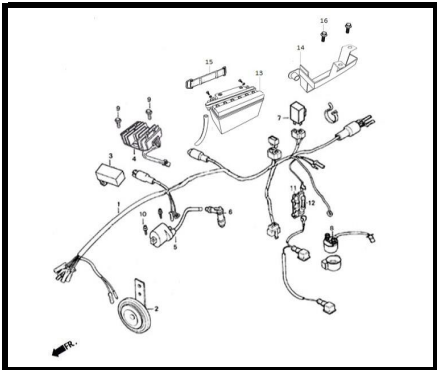
F-20 SISTEMA ELECTRICO
