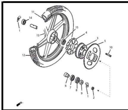
F-9 RUEDA TRASERA
