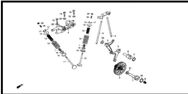
E-4-2 CILINDRO 150EVO
