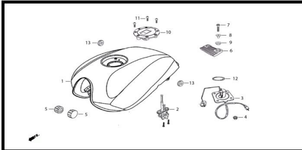
F-14 TANQUE COMBUSTIBLE
