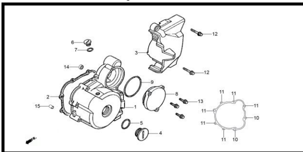
E-10 CARCAZAS CENTRALES
