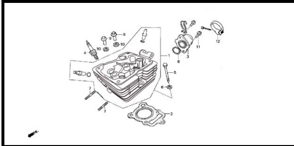
E-3-2 DISTRIBUCIÓN 150EVO
