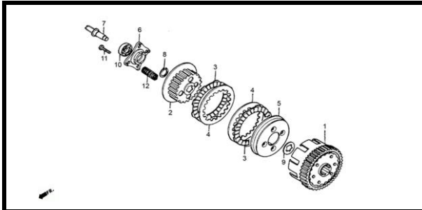
E-6 EMBRAGUE
