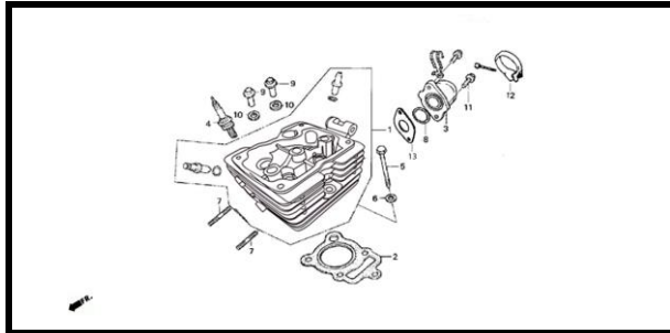
E-3-1 DISTRIBUCIÓN 125EVO
