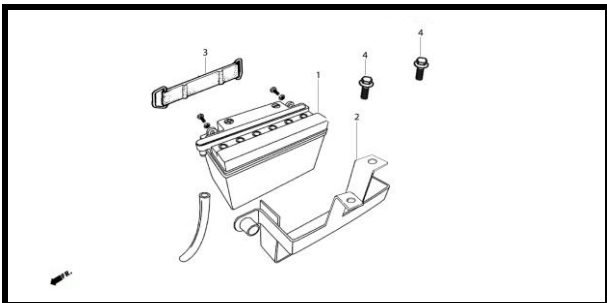
F-30 CHASIS
