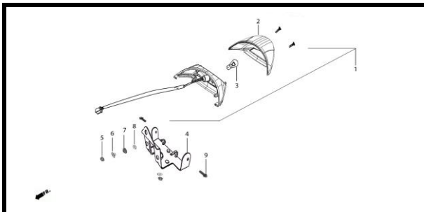
F-29 SISTEMA ELÉCTRICO
