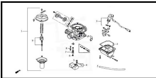
F-1-2 CARBURADOR 150 EVO 2009
