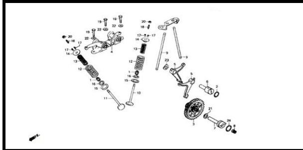
E-4-1 CILINDRO 125EVO
